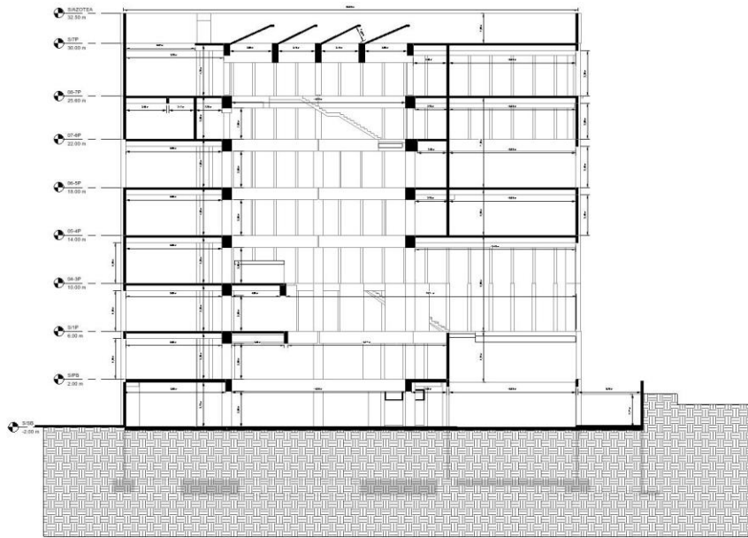
1 Seccion 1:100
