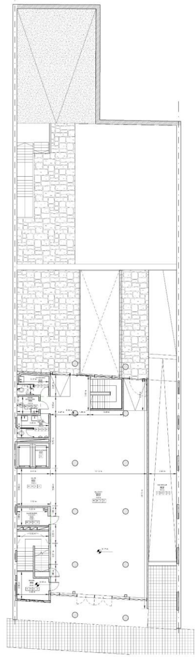
1 PLANTA BAJA 1 : 100
